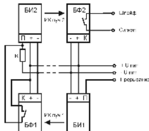
2-х лучевая ИК штора (схема подключения)
