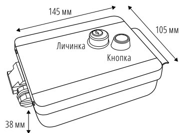
Рис. 1 Корпус замка
