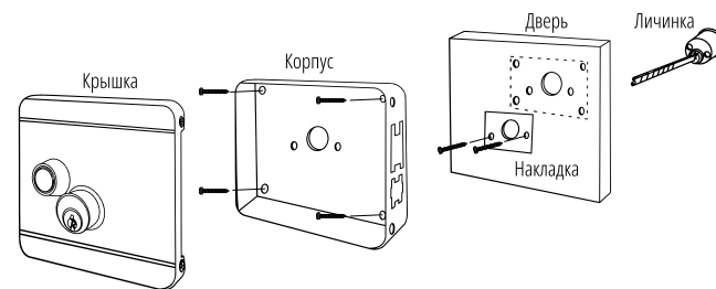
Рис. 4 Установка замка
