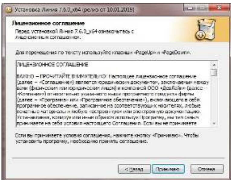
Рисунок 1.1 Лицензионное соглашение
