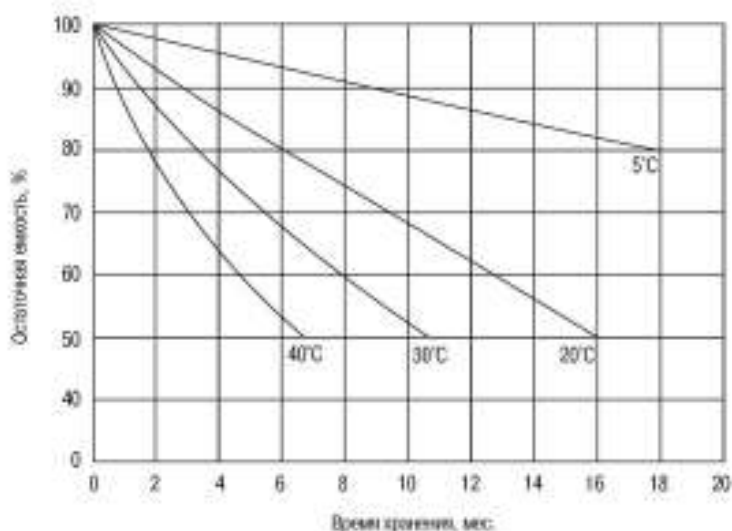
Рис. 9. Зависимость остаточной ёмкости от времени хранения при различных значениях температуры батареи.
