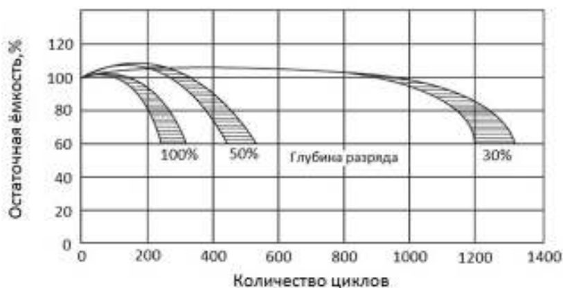
Рис. 8. Зависимость количества циклов от глубины разряда аккумуляторов серии «Болид».
