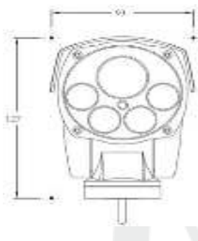
Рисунок 2. Внешние размеры (127х93мм)
