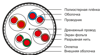
Рисунок 1 – Конструкция кабеля типа S/FTP
