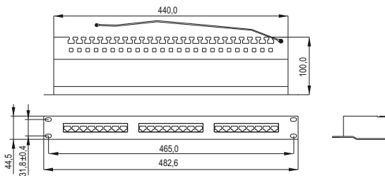
Рисунок/Figure 6 – PP24-1UC5ES-D05
