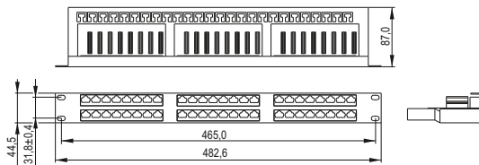
Рисунок/Figure 3 – PP48-1UC5EU-D05H
