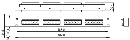
Рисунок/Figure 2 – PP24-1UC5EU-D05D
