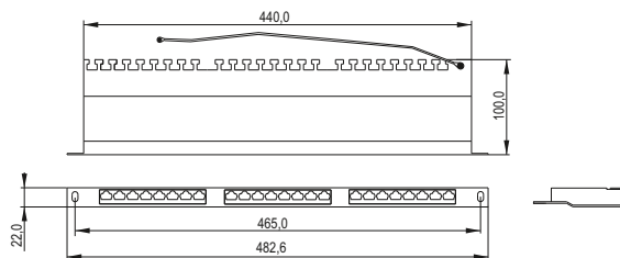
Рисунок/Figure 5 – PP24-D05UC5ES-D05H
