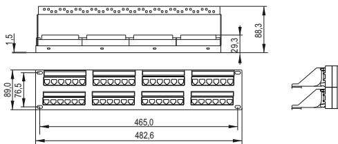
Рисунок/Figure 8 – PP48-2UC5EU-D05-1
