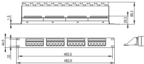
Рисунок/Figure 7 – PP24-1UC5EU-D05-1
