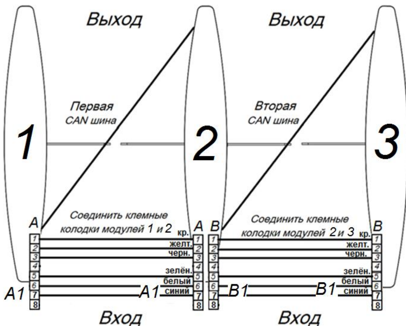
Рисунок 20 – Схема минимальных подключений для синхронной работы створок турникета
