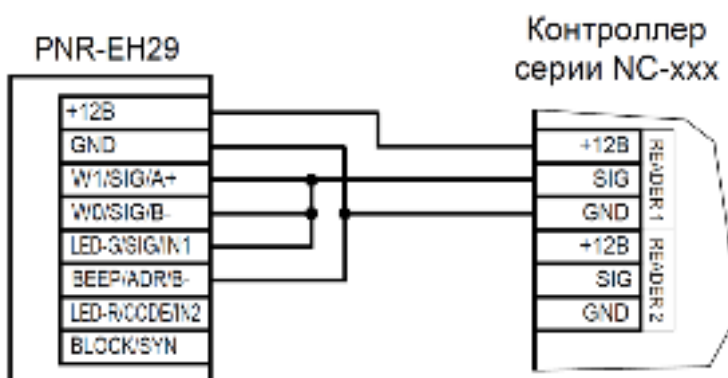
Рисунок 12. Подключение считывателя в режиме Parsec, адрес 0 (наружный)
