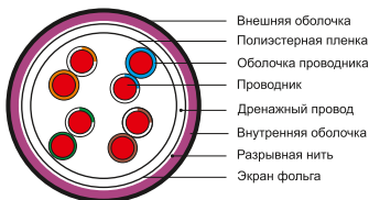
Рисунок 10 – Конструкция кабеля типа F/UTP (с двойной оболочкой)
