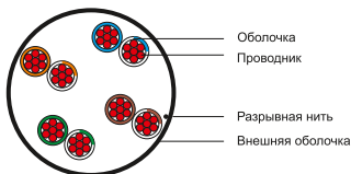
Рисунок 11 – Конструкция кабеля типа U/UTP (многопроводные жилы)
