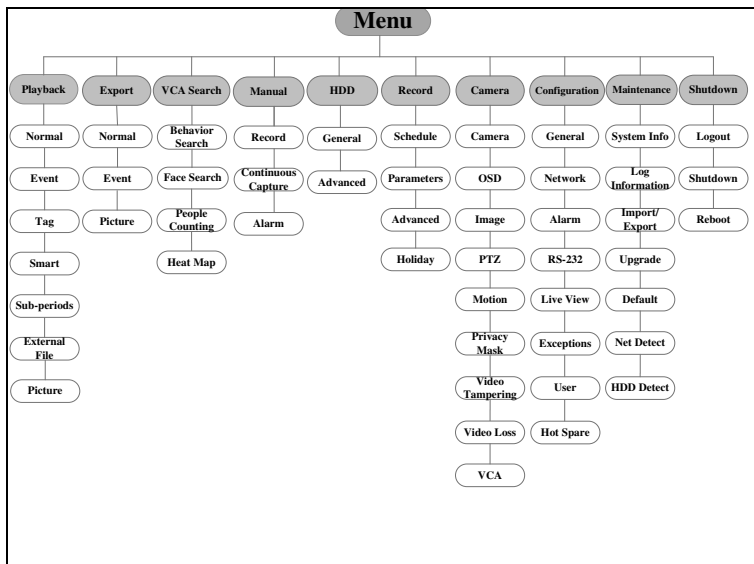
Рисунок 3.1 Структура меню
