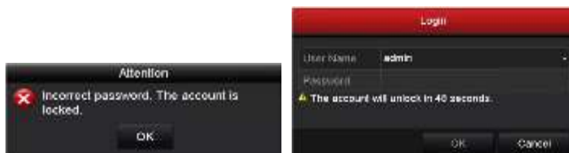
Рисунок 3.6 Блокировка аккаунта
