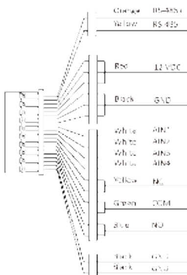
Рисунок 2-1. Описание разъемов
