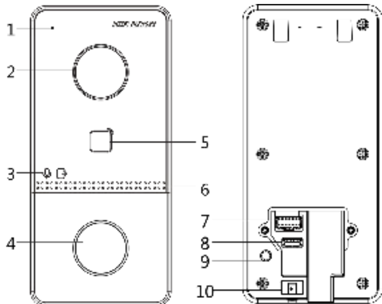
Рисунок 1-1. Передняя и задняя панели
