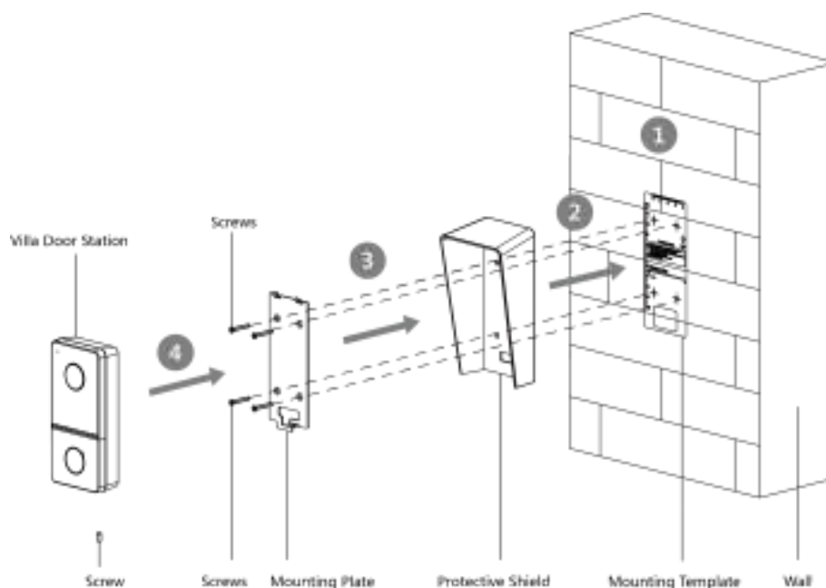
Рисунок 3-5. Врезная установка с защитным козырьком
