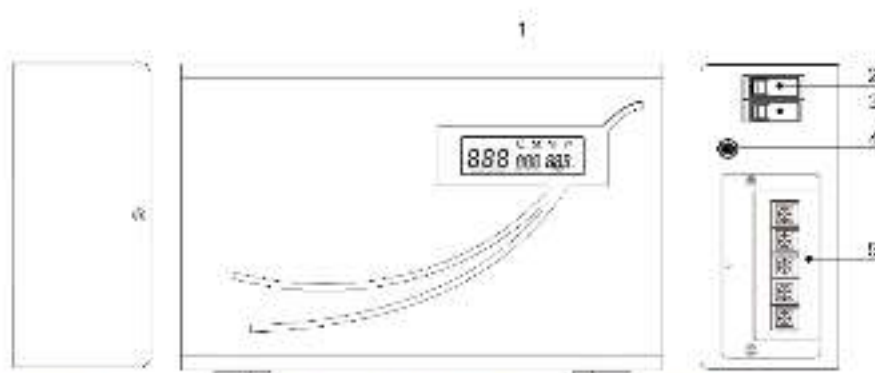
Рисунок 3. Внешний вид стабилизаторов напряжения SMARTWATT AVR SLIM 3000-5000VA. Описание элементов приводится в таблице 3.
