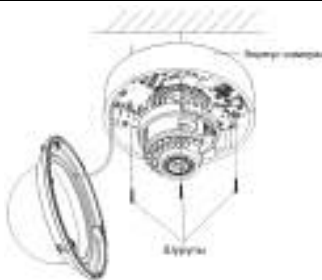
Рисунок 2-11 Установка камеры на потолок
