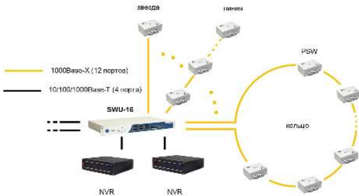
Рисунок 1.1 - Схема подключения
