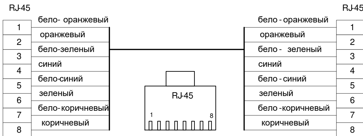
Рисунок 6.4 - Разделка кабеля.
