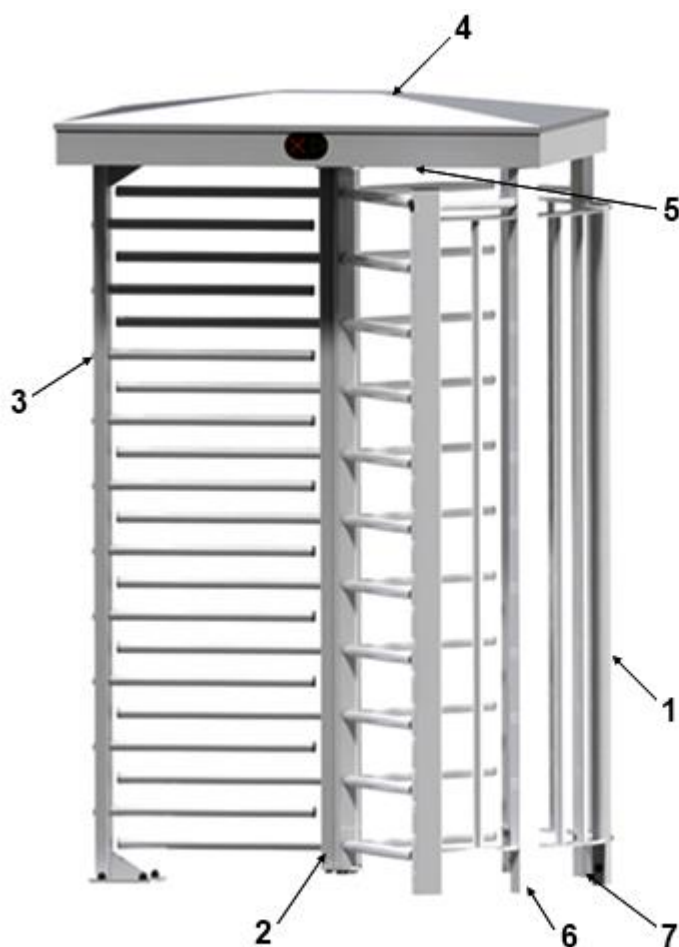
1 - неподвижная панель ограждения; 2 - роторная калитка 3 - неподвижные элементы ограждения; 4 - верхний модуль 5 - исполнительный механизм; 6,7 - стойка для подводки кабелей Рисунок 5 – Общий вид турникета
