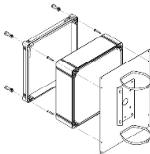
Рис.2. Монтаж кронштейна для крепления на квадратные и круглые опоры
