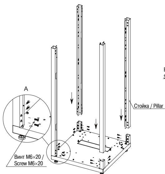
Рисунок 3 – Установка стоек / Figure 3 – Pillar installation
