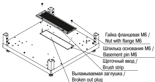
Рисунок 11 – Монтаж кабельного ввода / Figure 11 – Installation of brush strip
