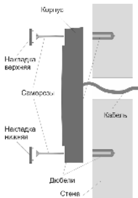
Рисунок 2. Крепление считывателя
