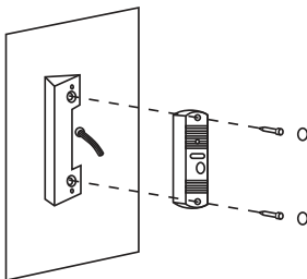
Рис. 6 Установка вызывной панели LEGEND под углом 30°.
