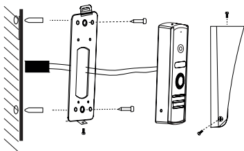
Рис. 7 Фронтальная установка вызывной панели MASK.
