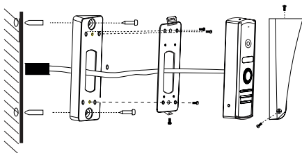
Рис. 8 Установка вызывной панели MASK под углом 30°.
