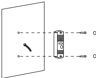
Рис. 5 Фронтальная установка вызывной панели LEGEND.
