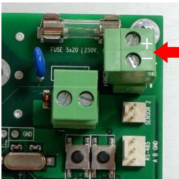
Рисунок 3.4.3 – Разъем для подключения альтернативного электропитания
