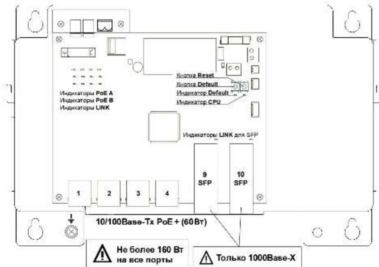
Рисунок 3.4.2 - Расположение элементов PSW-2G+VoX
