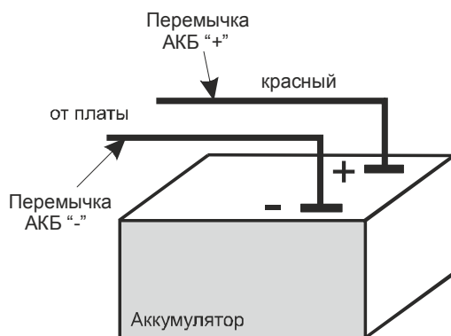
Рисунок 5. Подключение АКБ
