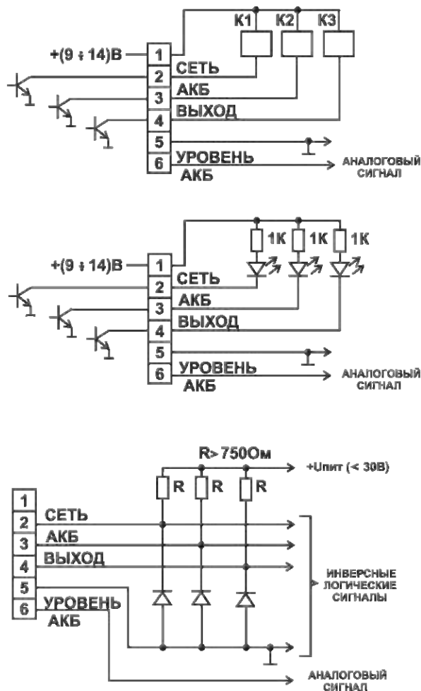
Рисунок 2. Примеры схем подключения исполнительных устройств к информационным выходам
