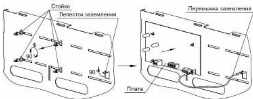
Рисунок 4. Установка платы
