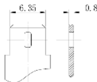
Клеммы
