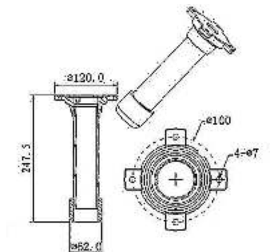
Рис. 2. Кронштейн крепления на горизонтальную поверхность
