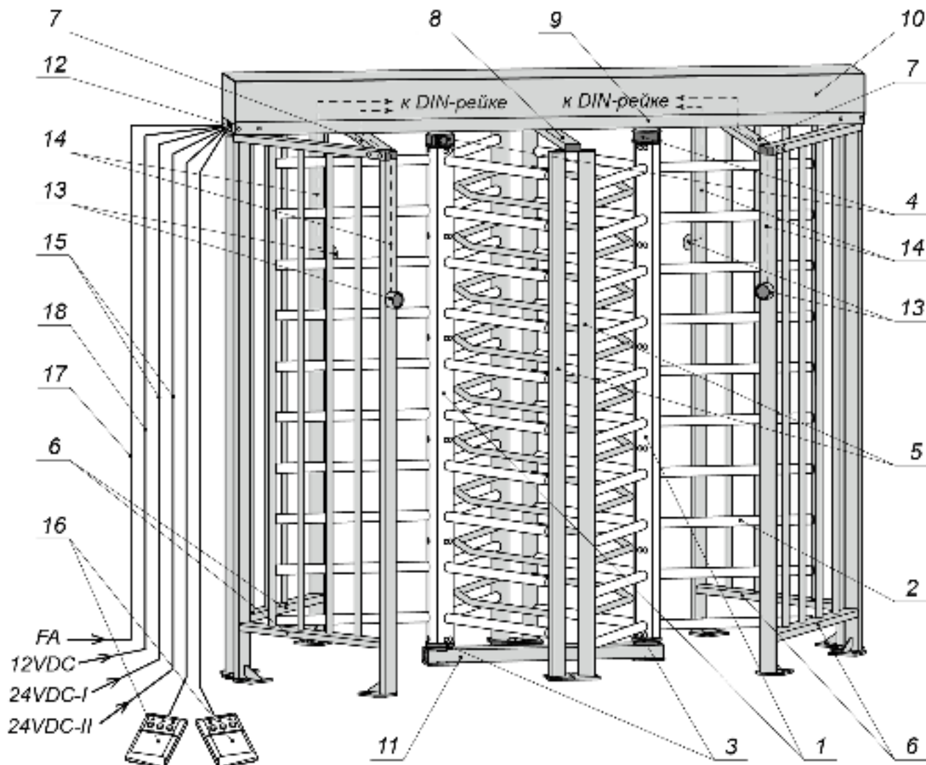
Рисунок 2. Устройство турникета:
