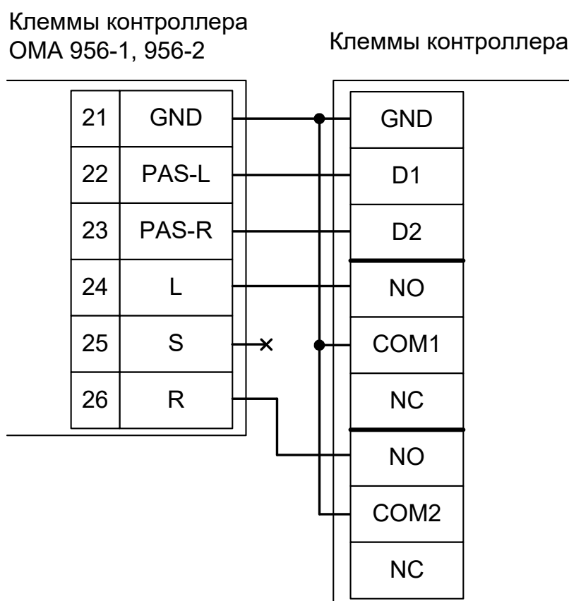
Рисунок 91. ОМА с контроллером ОМА 956-1, 956-2.
