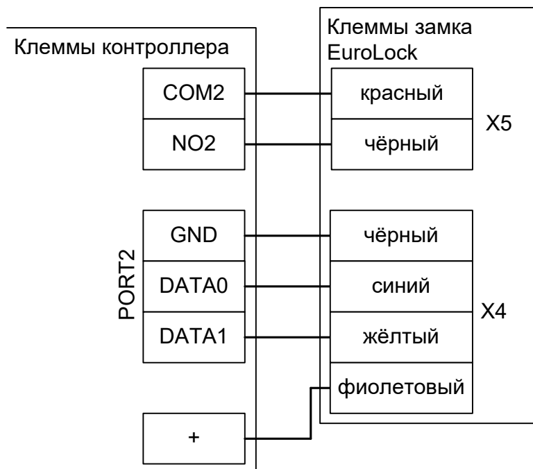
Рисунок 36. Пример подключения замка EuroLock ЕНТ на вход для первой двери.
