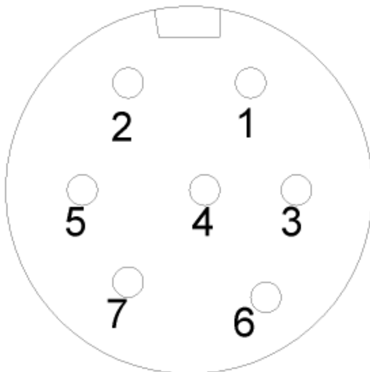
Рисунок 69. Разъём PC7.
