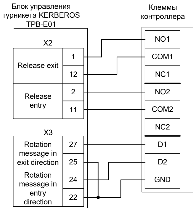
Рисунок 135. KABA Kerberos TPB-E01 с платой SINA 2.0.
