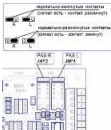
Рисунок 88. Перемычки JMP3 и JMP4 контроллера ОМА–DD.958, ОМА 264MC1, 866.MC2.
