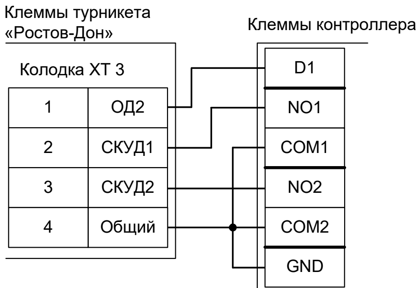
Рисунок 101. Турникеты и калитки «Ростов–Дон», старая электроника, вариант №1.
