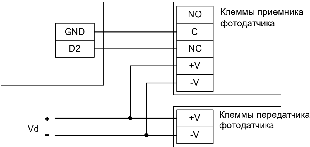
Рисунок 152. Пример подключение фотодатчика типа DOC на примере центрального датчика.
