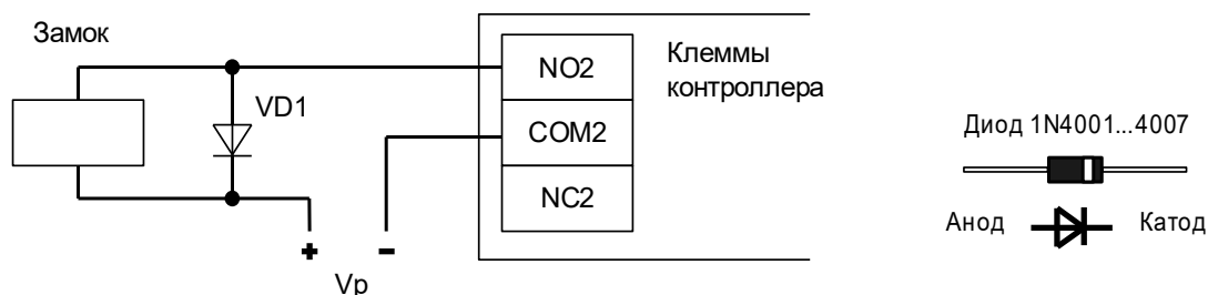
Рисунок 31. Пример подключения электромеханического замка для первой двери.
