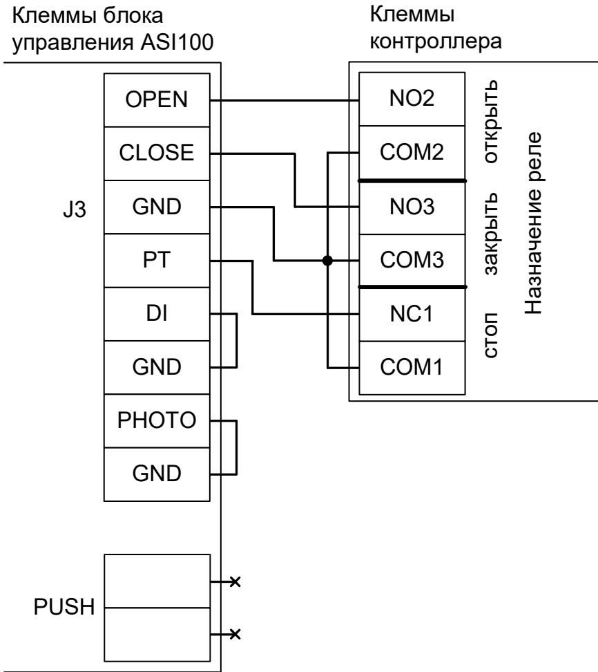
Рисунок 218. Подключение блока управления ворот ASI100.
