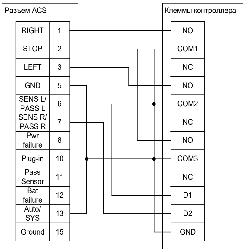
Рисунок 65. PERCo-TTR-04N и TTR-04W.
