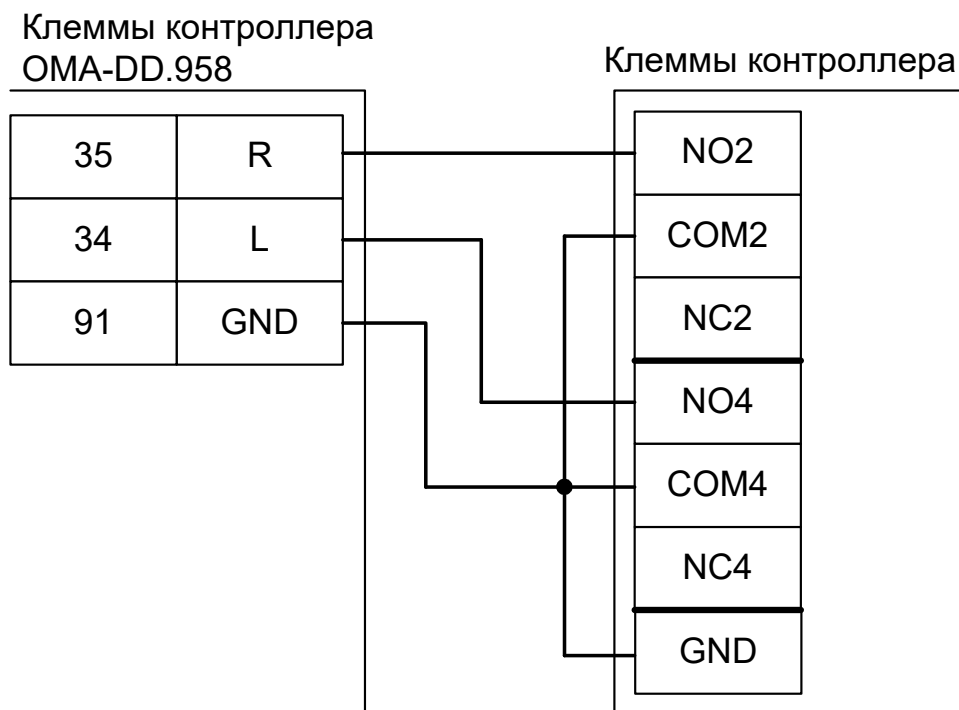
Рисунок 96. ОМА 36.68 с контроллером ОМА-DD.958.
