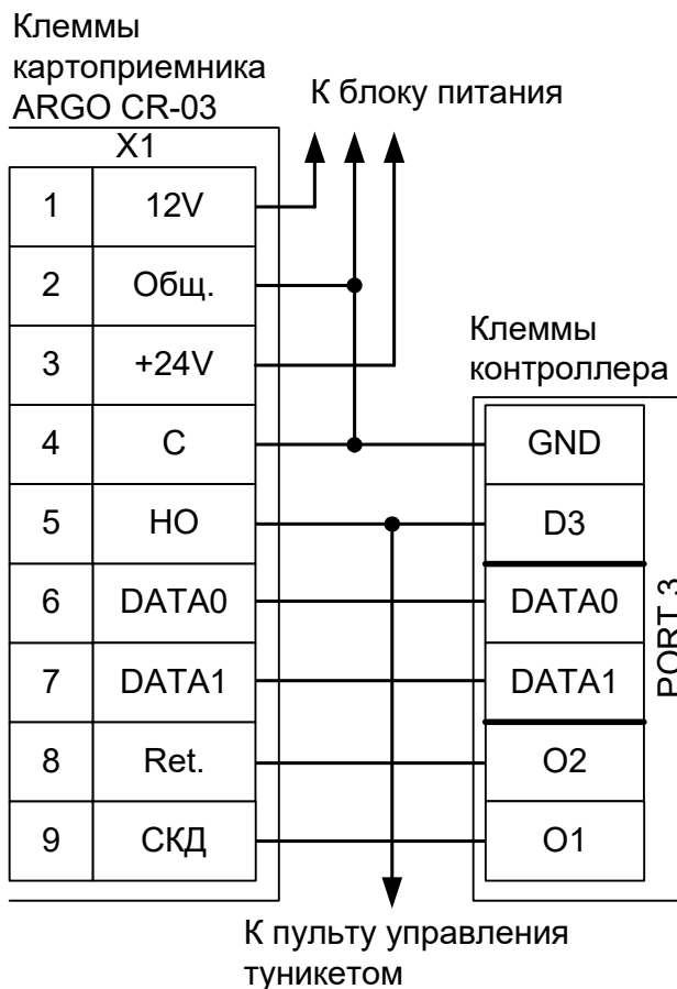
Рисунок 49. Пример подключения ARGO CR-03, TVER-7х в направлении «выход».
