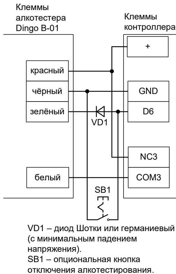
Рисунок 59. Вариант подключения Динго В-01 к турникету на вход.
