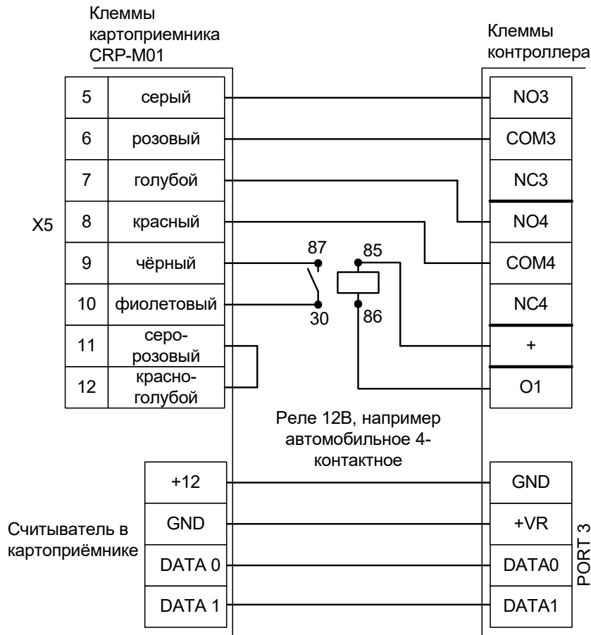
Рисунок 55. Пример подключения KABA CRP-M01.
