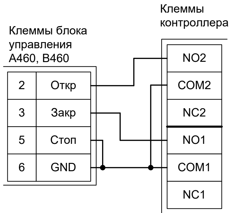
Рисунок 200. Hormann A460, B460.
