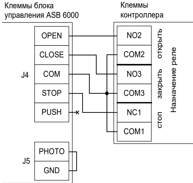
Рисунок 217. Подключение блока управления шлагбаума ASB6000.
