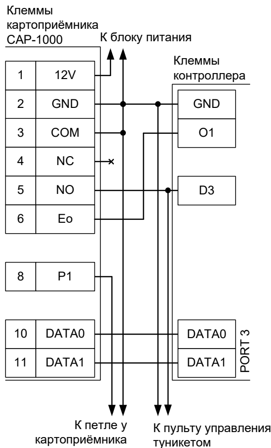
Рисунок 56. Пример подключения ParkFactor CAP-1000 в направлении «выход».
