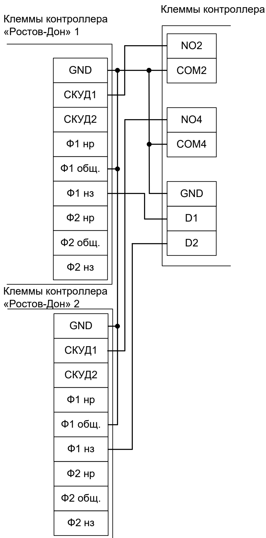
Рисунок 108. Двухпроходной турникет «Ростов-Дон».
