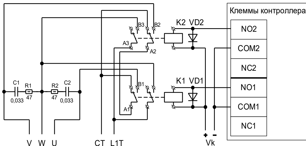
Рисунок 155. Подключение к мотор-редуктору FAST, KRONO, ATI, FERNI.
