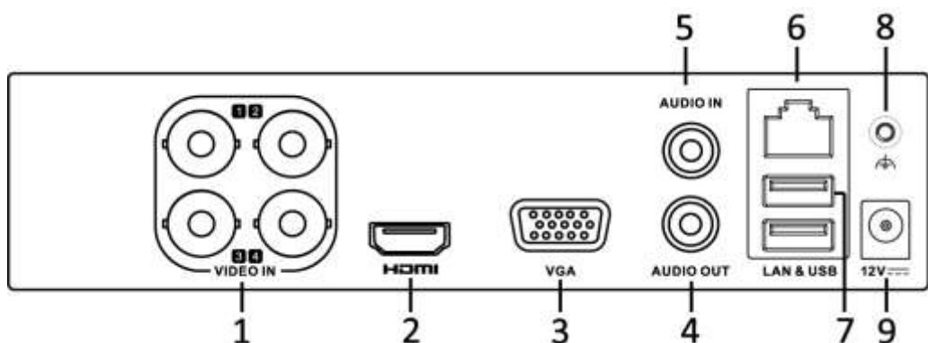
Рис. 1.2. Задняя панель регистратора LTV-RTB-040 00
