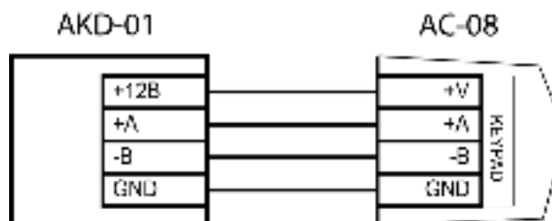
Рисунок 2. Схема подключения клавиатуры к охранному контроллеру
