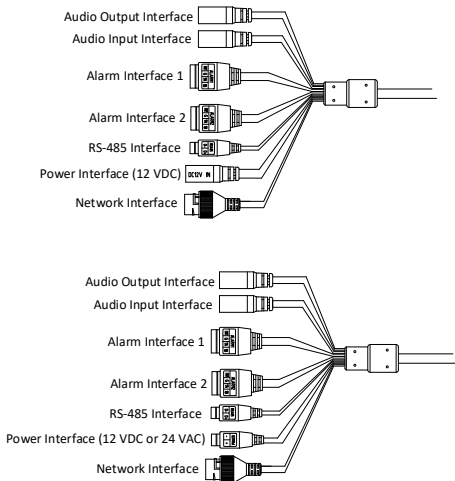
Рисунок 1-8 Описание кабелей
