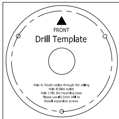
Рисунок 2-16 Шаблон крепления
