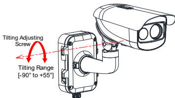
Рисунок 2-26 Регулировка по оси Т
