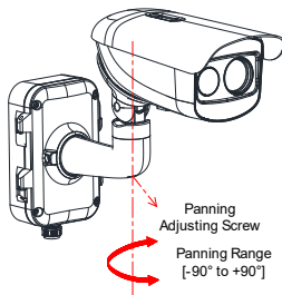
Рисунок 2-27 Регулировка по оси Р
