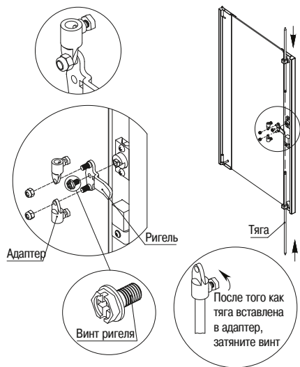
Рисунок 12 – Сборка дверей
