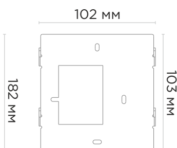
Кронштейн для накладного монтажа
