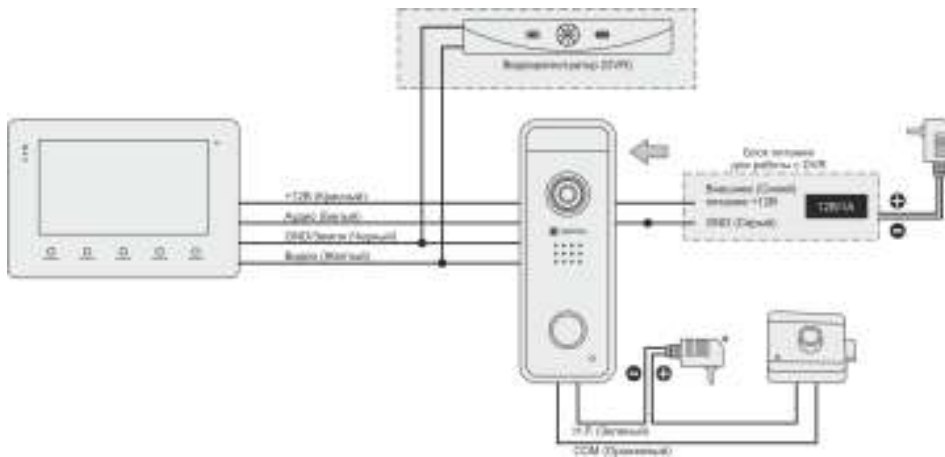
Рисунок 2. Схема подключения №2
