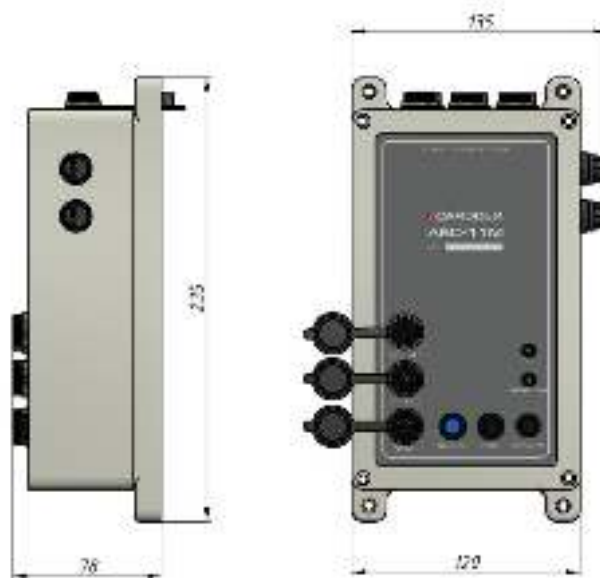
Рисунок 6.5.1.1 Габаритные размеры «ABC-11М»
