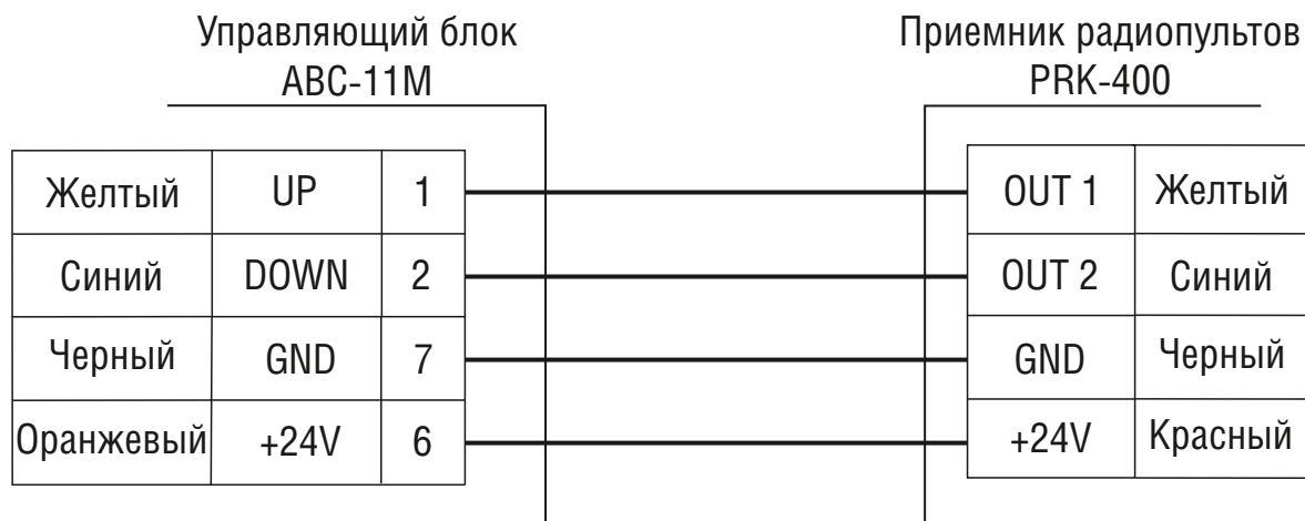
Рисунок 6.8.4 Схема подключения приемника радиопультов «PRK-400» к управляющему блоку «ABC-11M»
