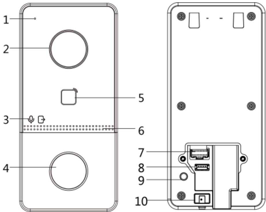
Рисунок 1-1. Передняя и задняя панели
