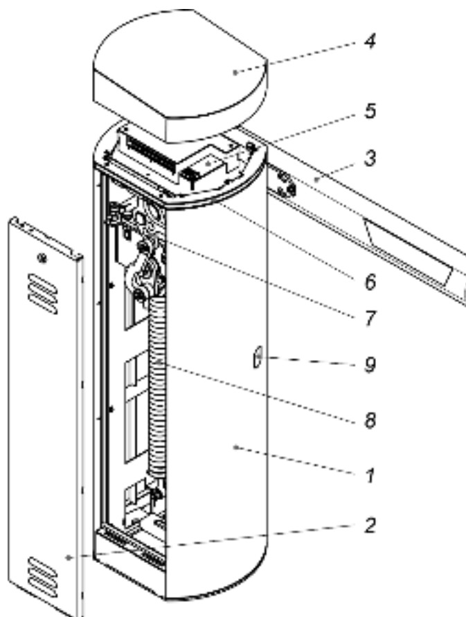
Рисунок 2. Устройство шлагбаума
