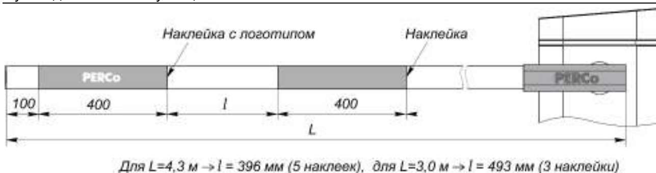
Рисунок 13. Наклеивание световозвращающих элементов на стрелу PERCo-GBR
