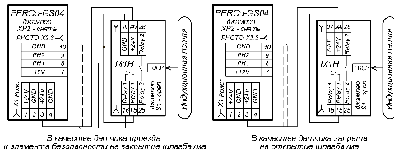
Рисунок 23. Варианты схемы подключения датчика индукционной петли к шлагбауму
