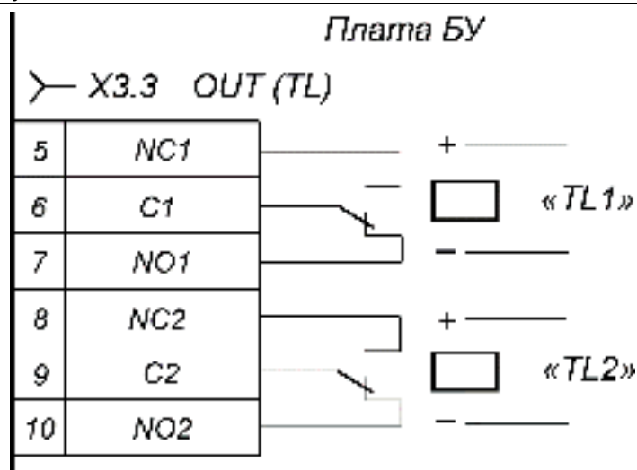
Рисунок 7. Выходные каскады для TL1, TL2
