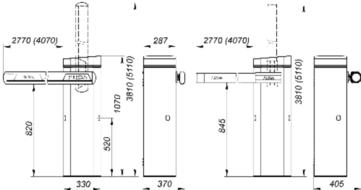
Рисунок 1. Габаритные размеры шлагдаума (вне скобок указаны размеры для стрелы длиной 3 м, в скобках для стрелы 4,3 м)
