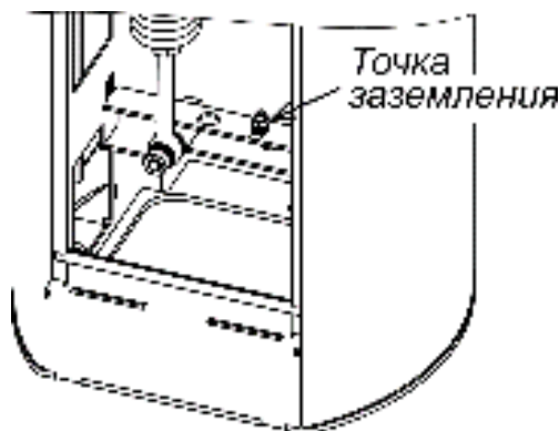
Рисунок 26. Расположение точки заземления шлагбаума
