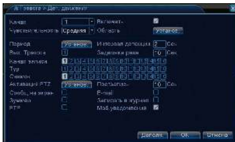
Обнаружение в гибридном (аналоговом) режиме
