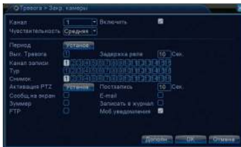
Заккрытие камеры в аналоговом режиме.
