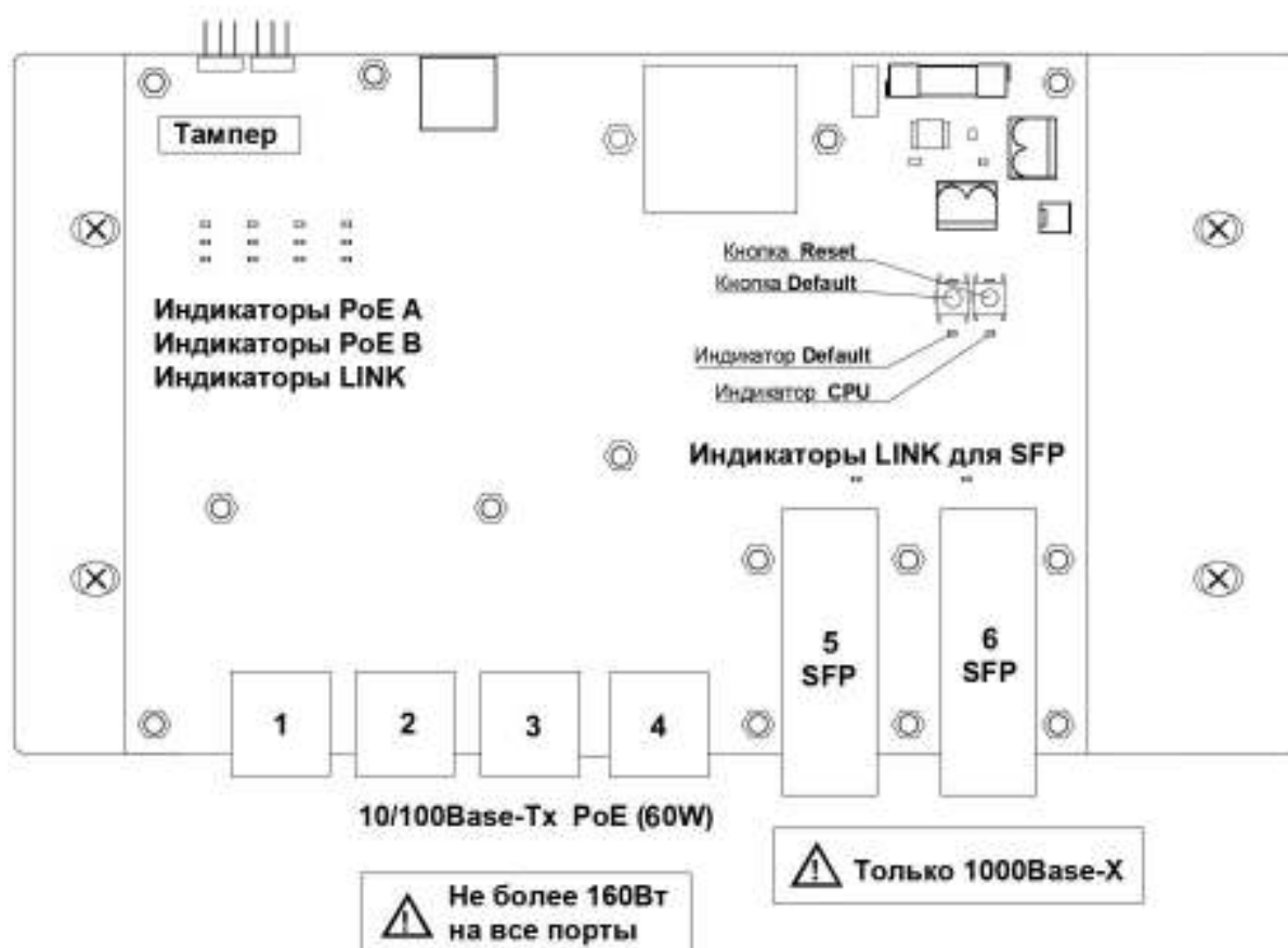
Рисунок 3.4.2 - Расположение элементов платы коммутатора
