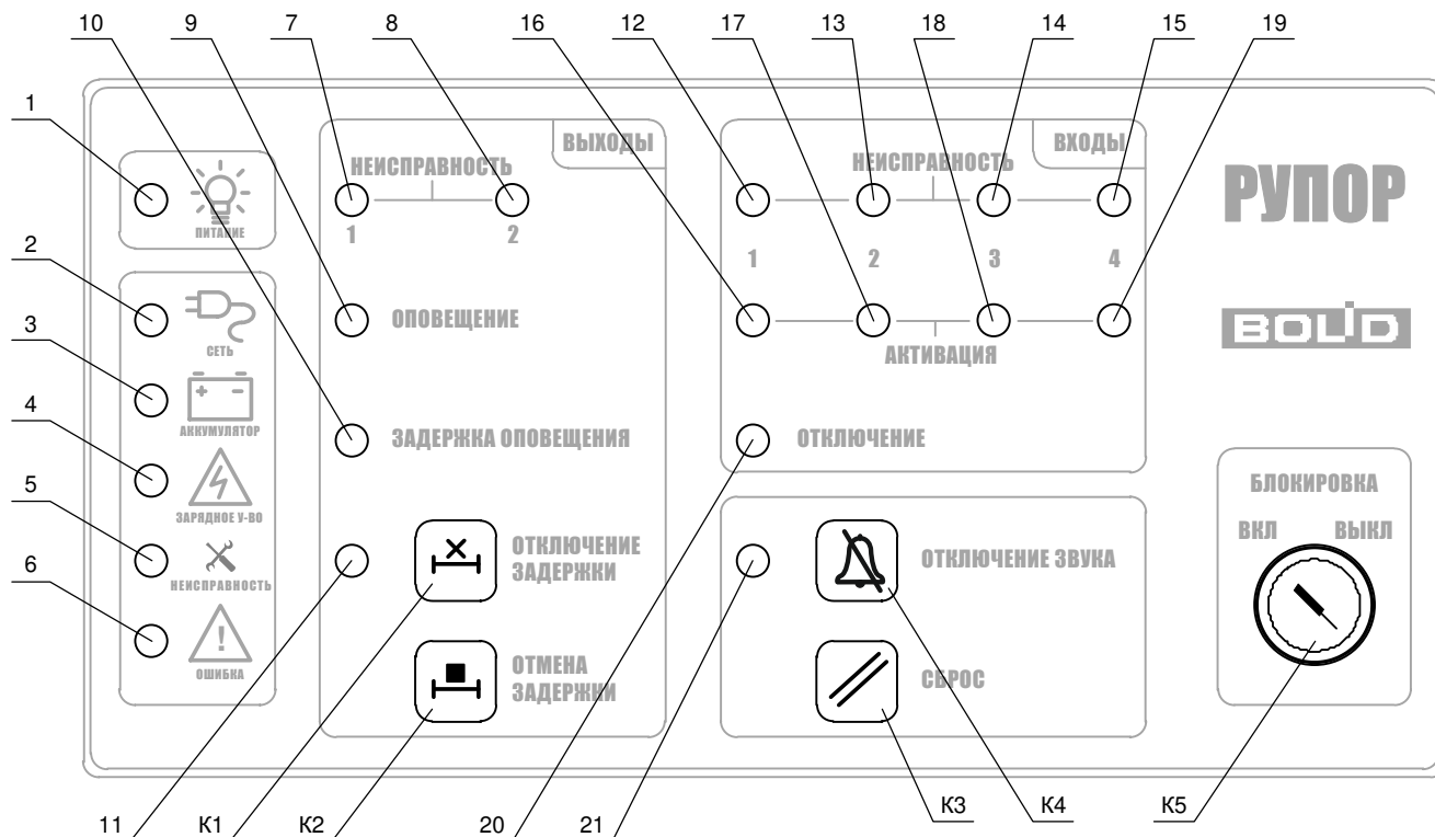
Рисунок 1. Органы управления и индикации блока
