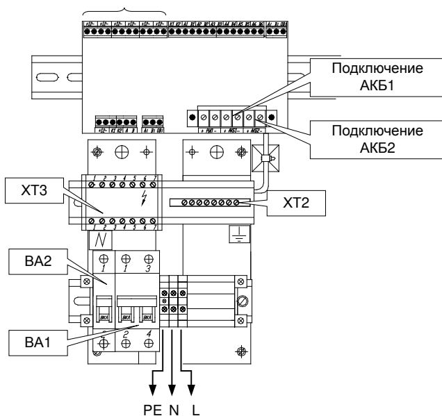
Рисунок 2 Схема расположения основных элементов «ШПС»
