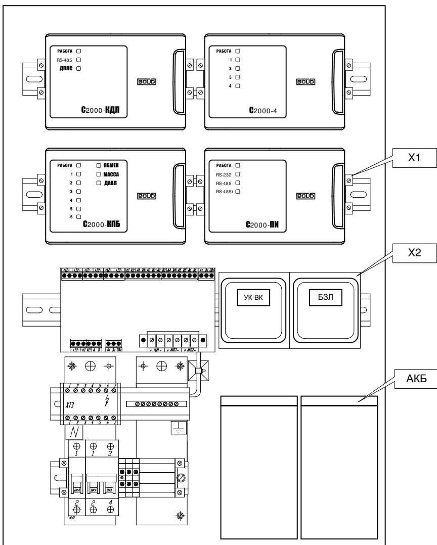
Рисунок 3 Пример компоновки «ШПС»
