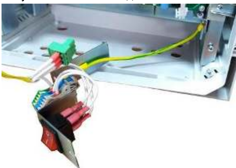
Рисунок 3.5.3 – Разъем питания 230 В отключен.
