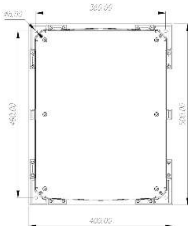
Рисунок 7.2 - Разметка крепления
