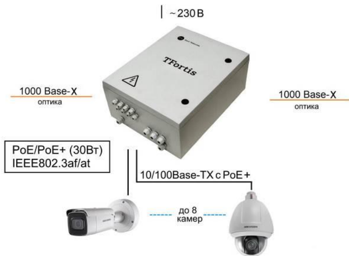
Рисунок 1 - Схема подключения PSW-2G8F+UPS-Box
