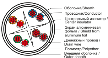
Рисунок 4 - Конструкция патч-корда категории 6 типа F/UTP / Figure 4 - Design of F/UTP patch cord of 6 category
