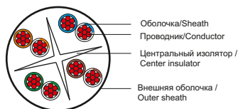
Рисунок 3 - Конструкция патч-корда категории 6 типа U/UTP / Figure 3 - Design of U/UTP patch cord of 6 category
