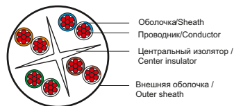
Рисунок 5 - Конструкция патч-корда категории 6A типа U/UTP / Figure 5 - Design of U/UTP patch cord of 6A category
