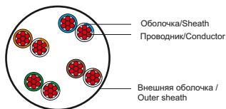
Рисунок 1 - Конструкция патч-корда категории 5е типа U/UTP / Figure 1 – Design of U/UTP patch cord of 5e category
