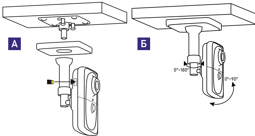
Рис. 13 Установка видеокамеры PRO ×05
