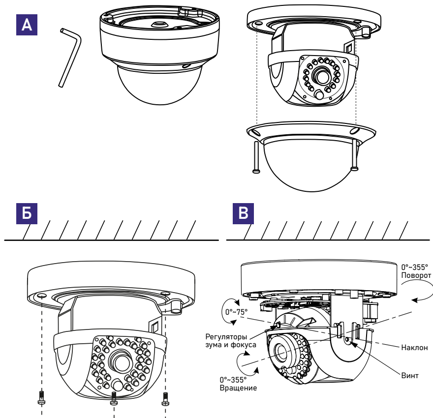
Рис. 14 Установка видеокamеры PRO x07
