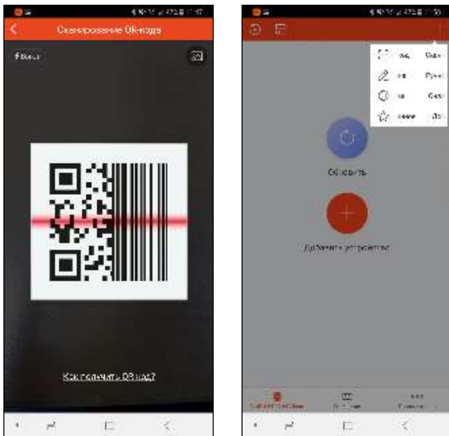
Рис. 36 Добавление устройства-2
