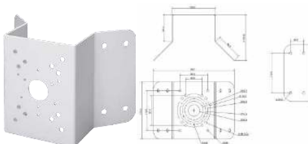
Рисунок 5.7 – Угловой кронштейн BR-102
