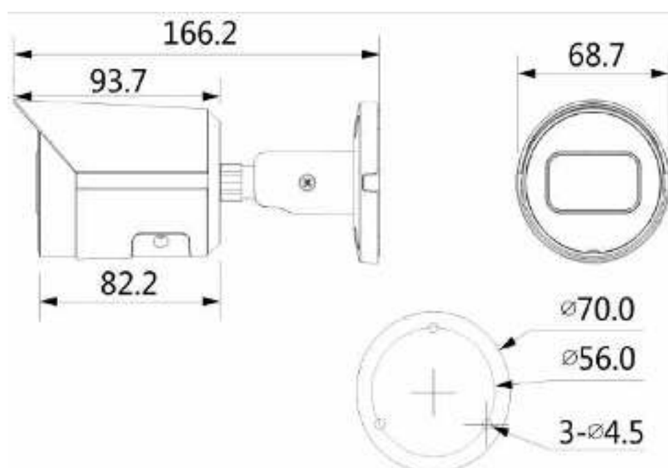
Рисунок 5.1 – Габаритные размеры видеокамеры
