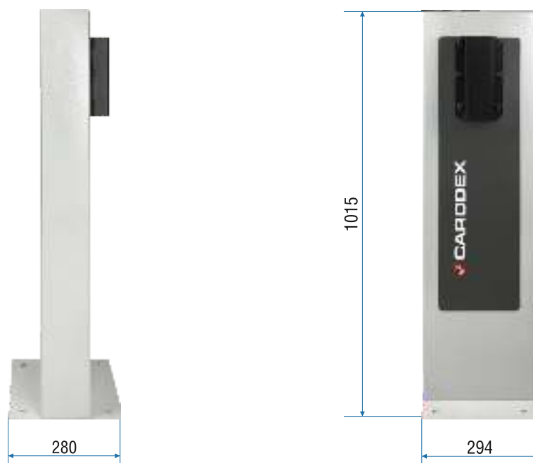
Рисунок 4.1. Габаритные размеры тумбы шлага.
