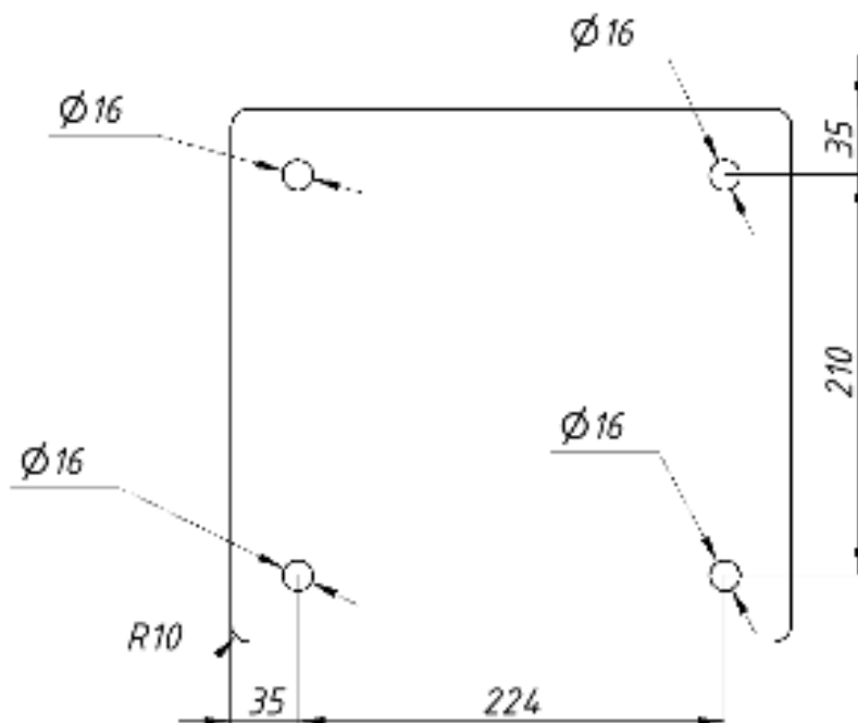
Рисунок 6.4.2. Монтажное основание.
