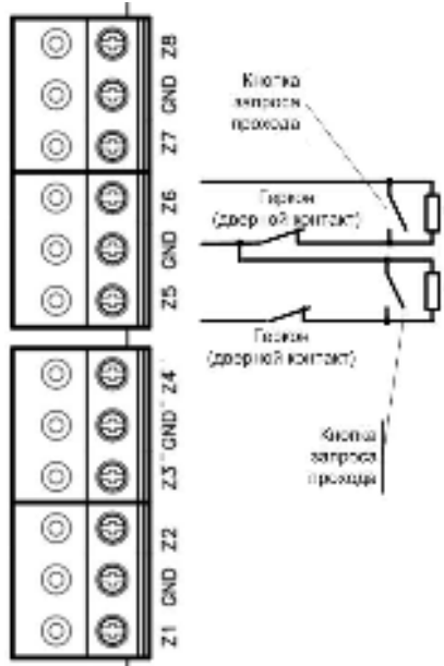
Рис.14. Подключение комбинированного шлейфа
