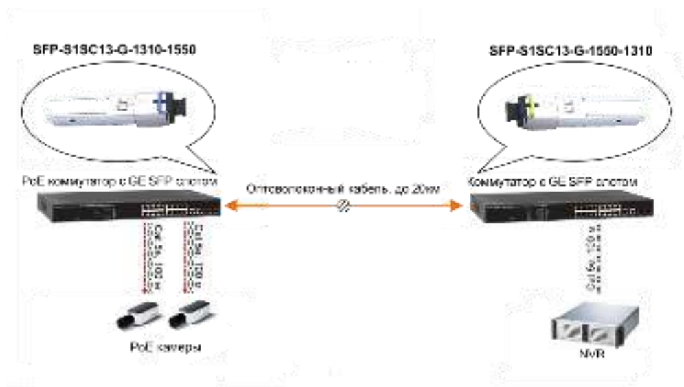
Рис.6 Типовая схема подключения SFP модулей SFP-S13C13-G-1310-1550, SFP-S13C13-G-1550-1310
