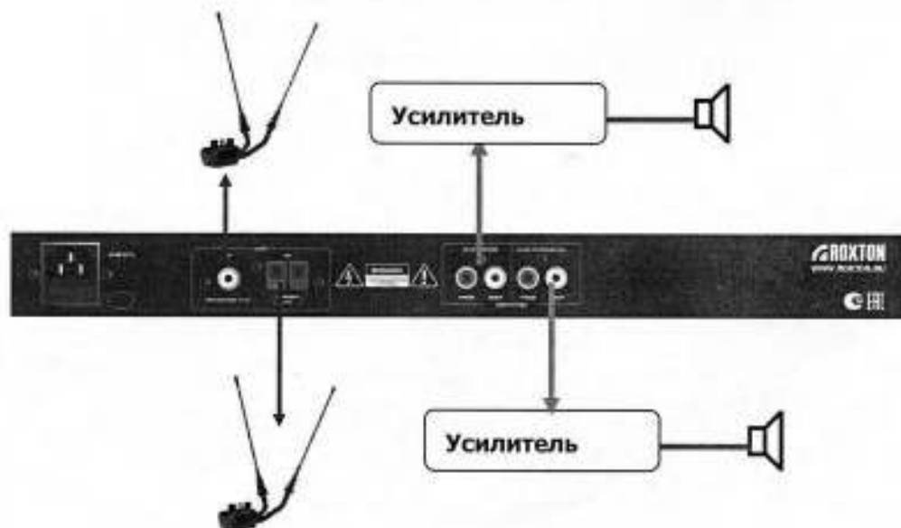
Типовая схема подключения
