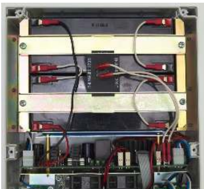
Рис. 2.9.5. Подключение АКБ.
