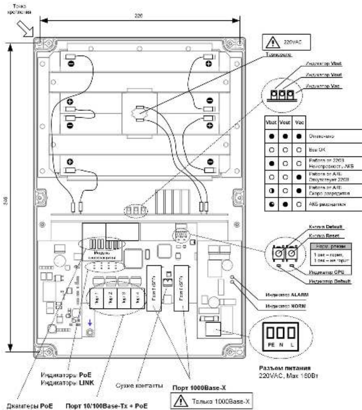
Рис. 2.2-2. Расположение элементов PSW -2G4F-UPS
