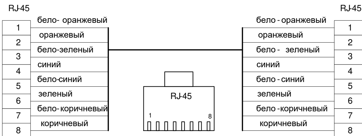
Рис. 6.4. Разделка кабеля.
