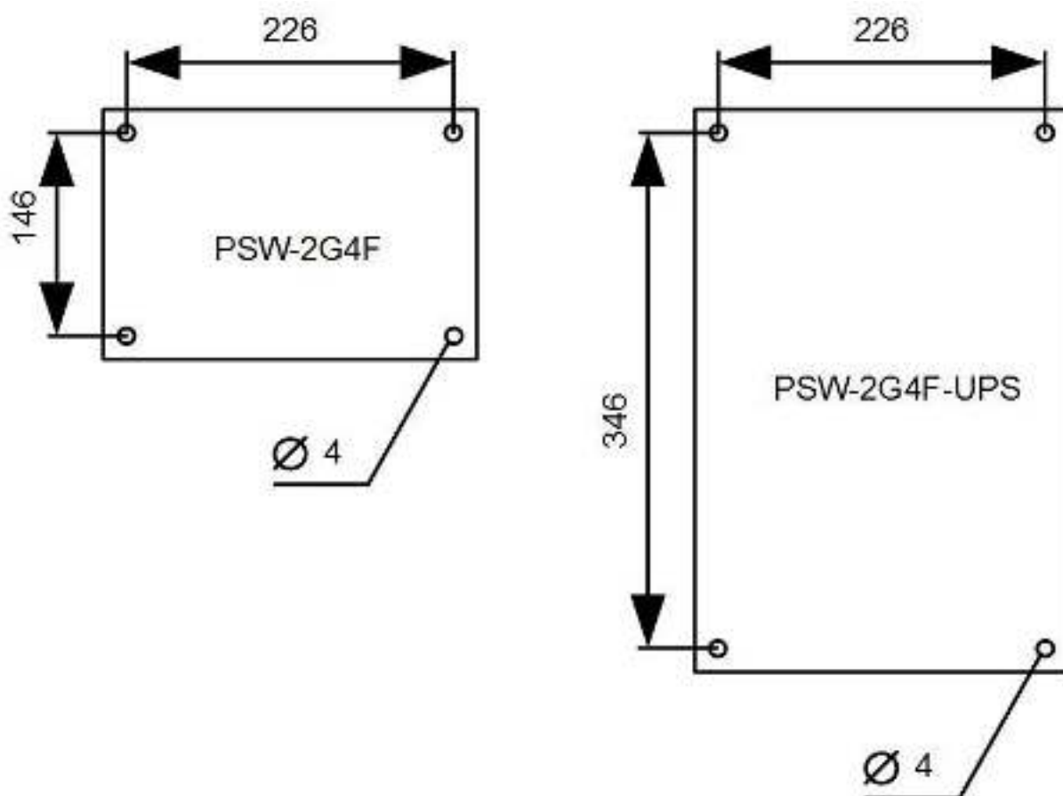
Рис. 6.1.1. Разметка крепления
