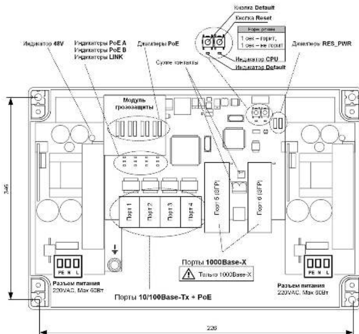
Рис. 2.2-1. Расположение элементов PSW -2G4F
