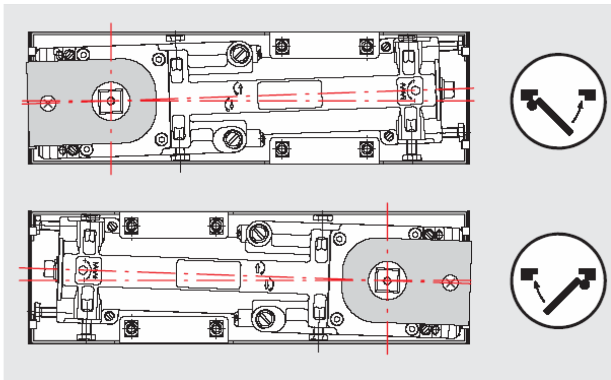
Рис. 11. Второй вариант установки напольного доводчика DORMA BTS75V болтового крепления.
