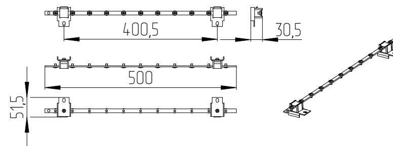
Панель заземления ПЗ-500.80А (ПЗ-500.200А)
