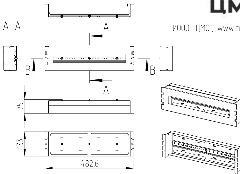
Панель 19" с DIN-рейкой КП-AB
