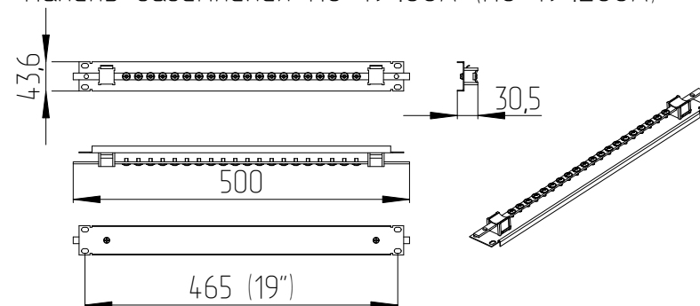
Панель заземления ПЗ-19".80А (ПЗ-19".200А)
